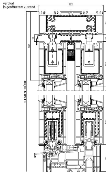
Darstellung Schwelle GU-934 K
