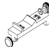
628 420 HST - Bohrerschablone (GU-Schwelle 934 K) (Siegeniaschwelle 300 KF)
